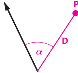
Polar coordinates
