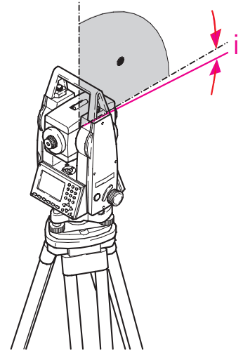
Height-index error (i) (V index)
